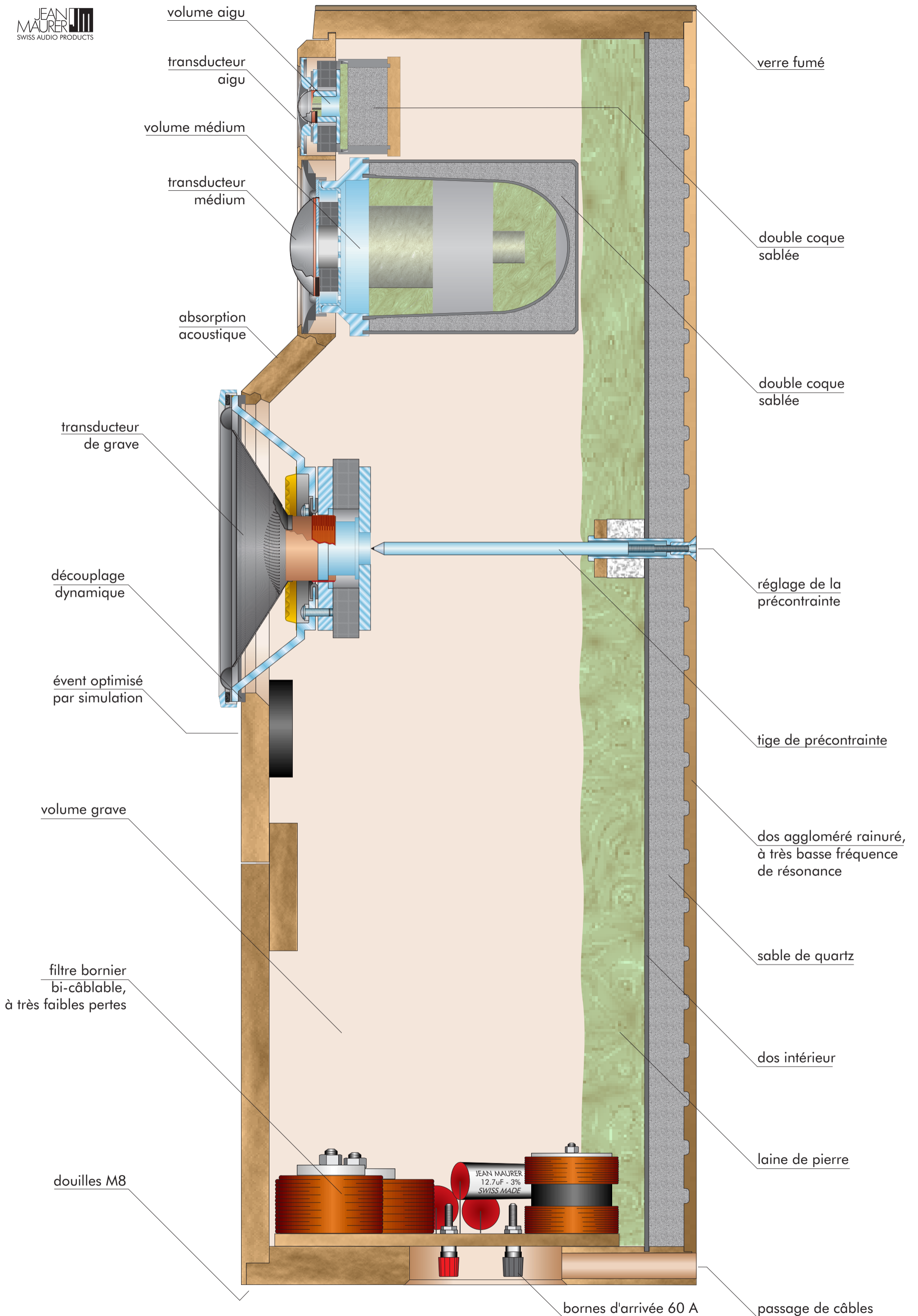
Enceinte acoustique Jean Maurer 370 E
